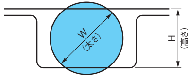
図1-2 Oリングの使い方
